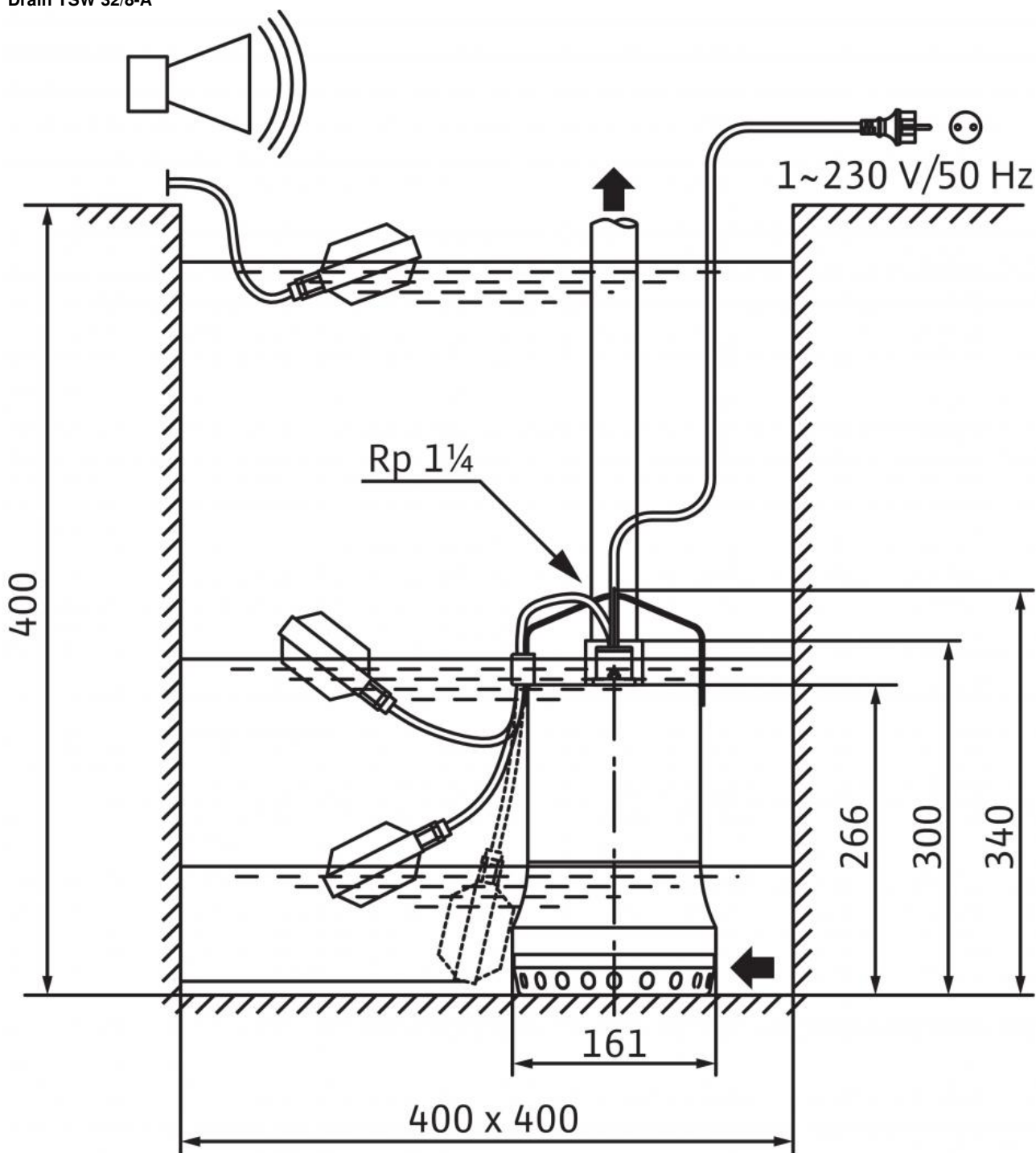
Rozmerový výkres Drain TSW 32/8-A
