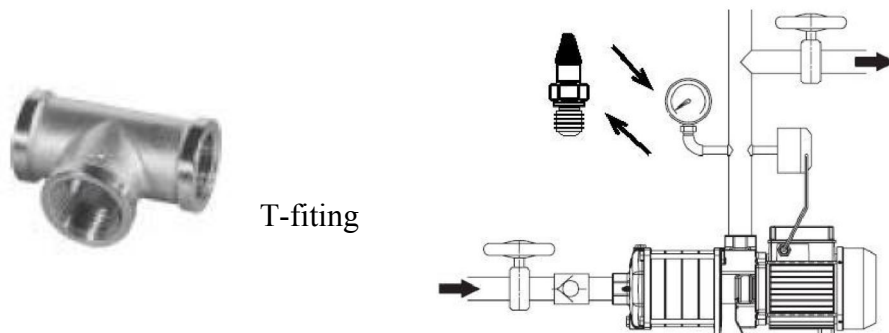
Obr. 6: Výmena TS za manometer
