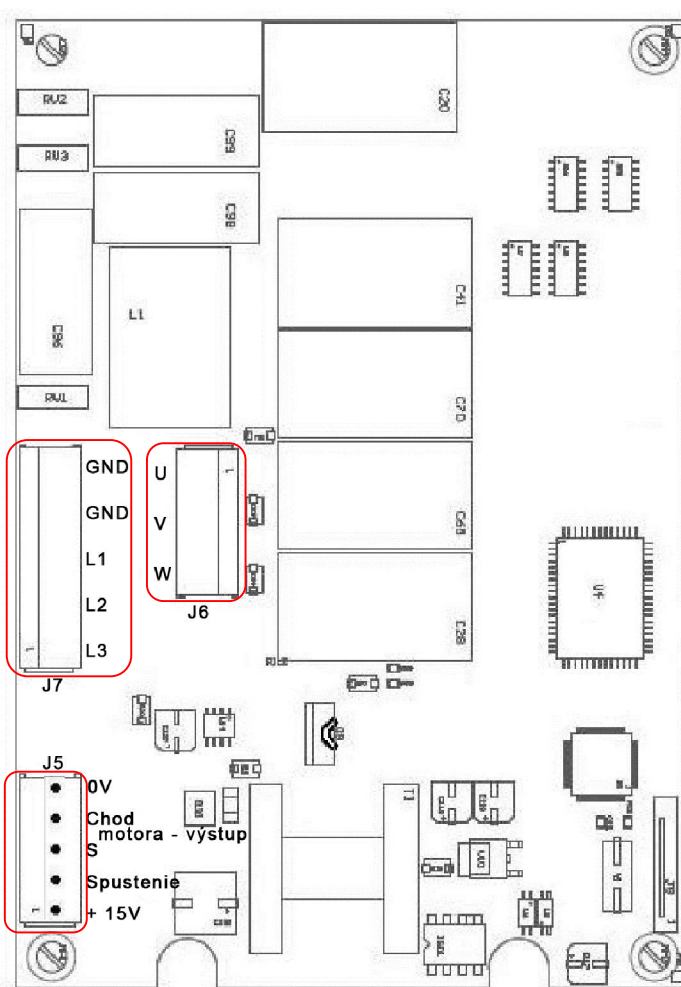
Obr.14: Elektronická doska ITTP1.W-BC
