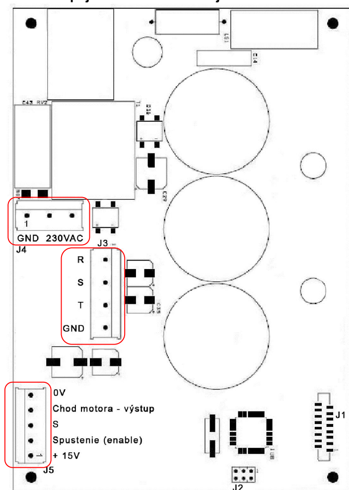
Obr.13: Elektronická doska IMMP-IMTP1.5W-BC
