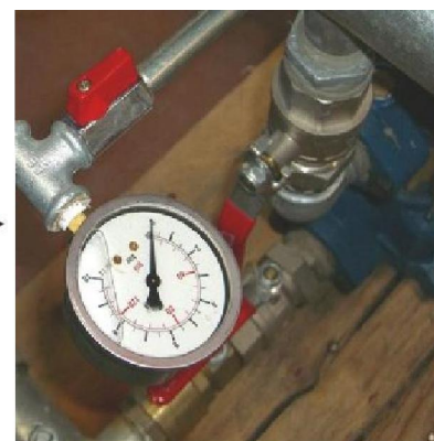
Obr. 6: Výmena TS za manometer
