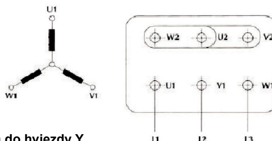
Obr. 12 – Zapojenie motora do hviezdy Y
