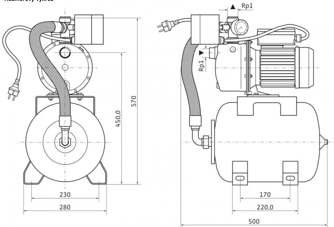
Rozmerový výkres
