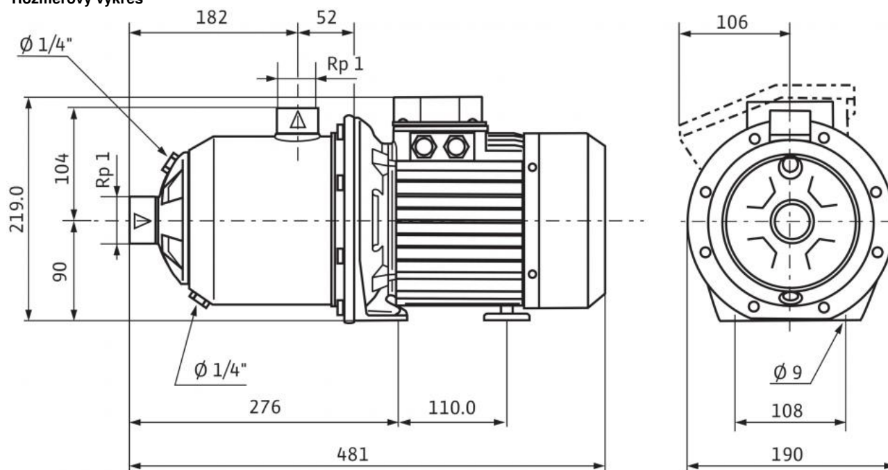
Rozmerový výkres
