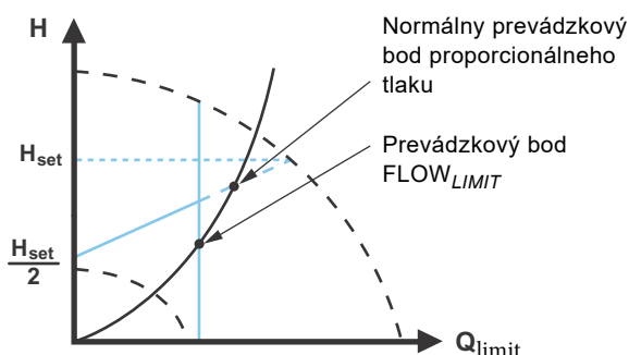
Obr. 39 Riadenie podľa proporcionálneho tlaku s FLOW LIMIT
