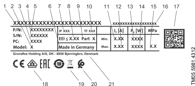
Obr. 19 Príklad typového štítku
