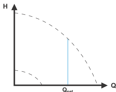
Obr. 35 Konštantný prietok
