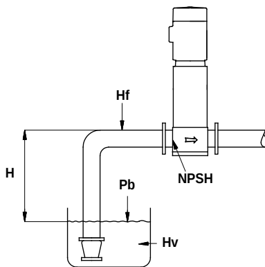
Obr. 21 Schematické znázornenie otvorenej sústavy s čerpadlom CR
