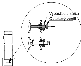
Obr. 18 Umiestnenie vypúšťacej zátky a obtokového ventilu
