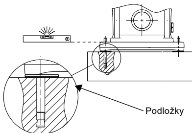
Obr. 6 Vyrovnanie pomocou podložiek
