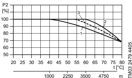
Obr. 19 Výkon motora v súvislosti s teplotou a nadmorskou výškou
