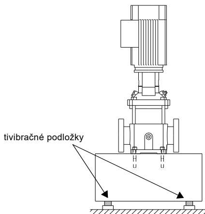
Obr. 7 Čerpadlo na antivibračných podložkách
