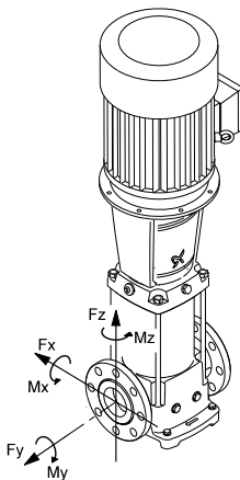
Obr. 9 Sily a uťahovacie momenty na prírubе
