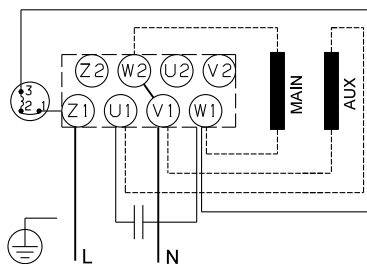
Obr. 12 Pripojenie, 220-230 V, 0,37 - 0,75 kW
