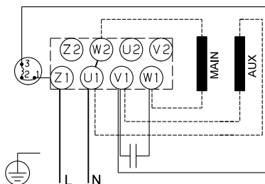
Obr. 13 Pripojenie, 240 V, 0,37 - 0,75 kW
