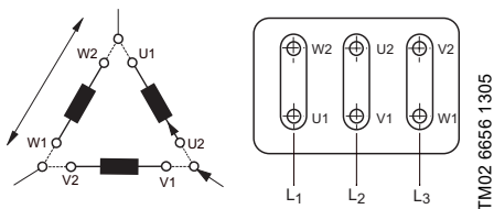
Obr. 10 Zapojenie do trojuholníka
