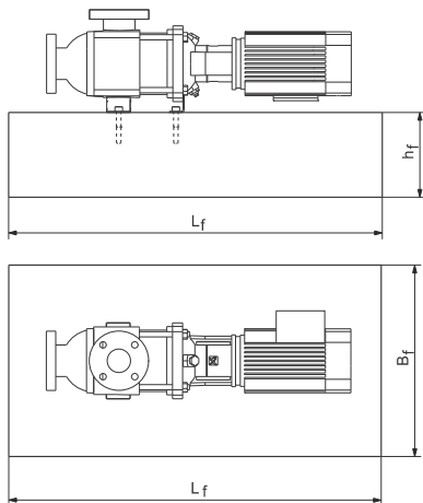
Obr. 4 Základňa, horizontálna montáž
