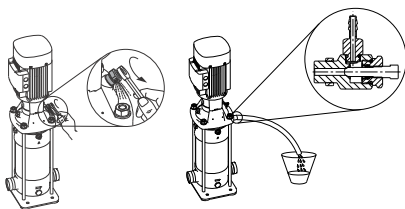
Obr. 16 Odvzdušňovací ventil, štandardné a voliteľné riešenie s pripojením hadice
