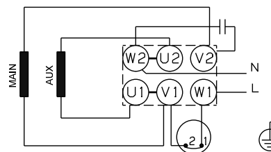
Obr. 15 Pripojenie, 240 V, 1,1 - 2,2 kW
