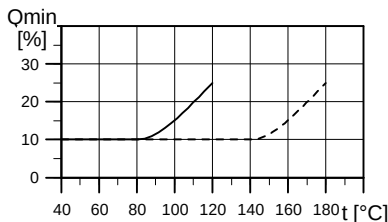
Obr. 22 Minimálny prietok
