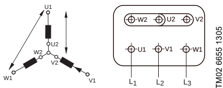
Obr. 11 Zapojenie do hviezdy
