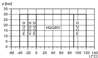
Obr. 20 Maximálny prípustný prevádzkový tlak a teplota čerpanej kvapaliny
