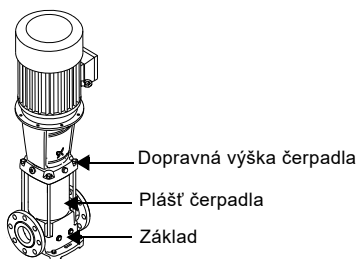
Obr. 17 Horúce alebo studené povrchy na čerpadle CR, CRI a CRN
