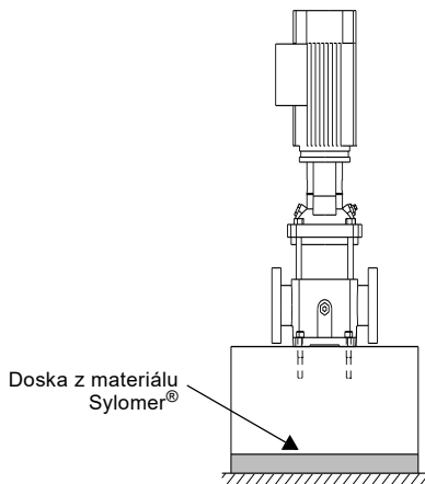
Obr. 8 Čerpadlo na doske z materiálu Sylomer®
