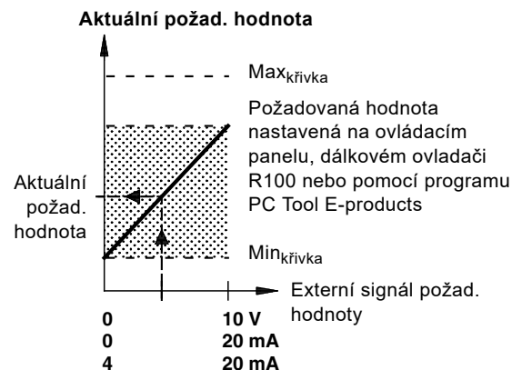
Obr. 31 Vztah mezi aktuální požadovanou hodnotu a signálem externí požadované hodnoty v neregulovaném řídicím režimu
