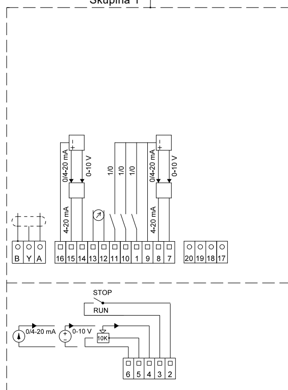
Obr. 10 Připojovací svorky rozšiřovacího I/O modulu
