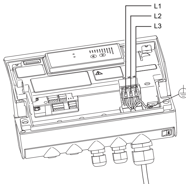
Obr. 3 Síťová přípojka
