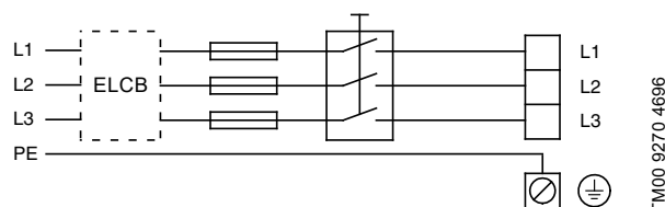
Obr. 6 Čerpadlo připojené na přívod napájecího napětí s hlavním spínačem, záložní pojistkou, přídavnou ochranou a ochranným uzemněním
