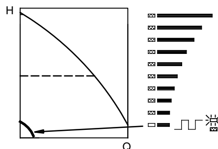
Obr. 18 Provoz podle min. křivky
