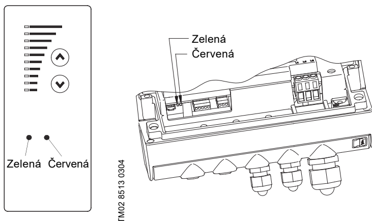
Obr. 33 Polohy signálních světel u třífázových čerpadel
