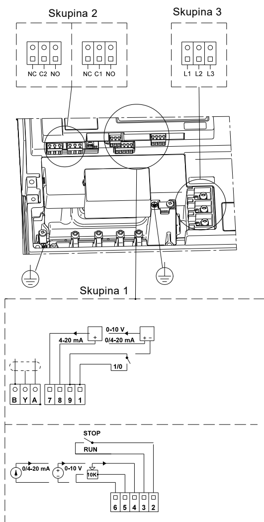
Obr. 5 Připojovací svorky I/O modulu čerpadla
