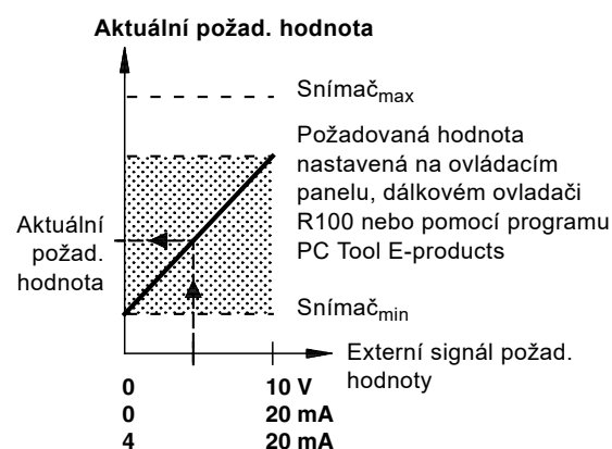
Obr. 30 Vztah mezi aktuální požadovanou hodnotu a signálem externí požadované hodnoty v regulovaném řídicím režimu
