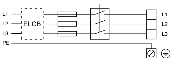
Obr. 2 Čerpadlo připojené na přívod napájecího napětí s hlavním spínačem, záložní pojistkou, přídavnou ochranou a ochranným uzemněním
