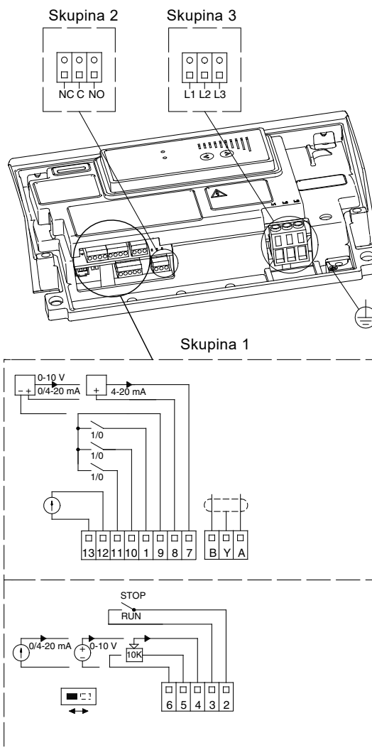
Obr. 4 Připojovací svorky rozšiřovacího I/O modulu
