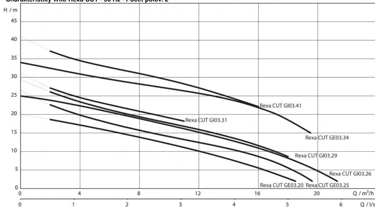
Charakteristiky Wilo-Rexa CUT - 50 Hz - Počet pólov: 2
