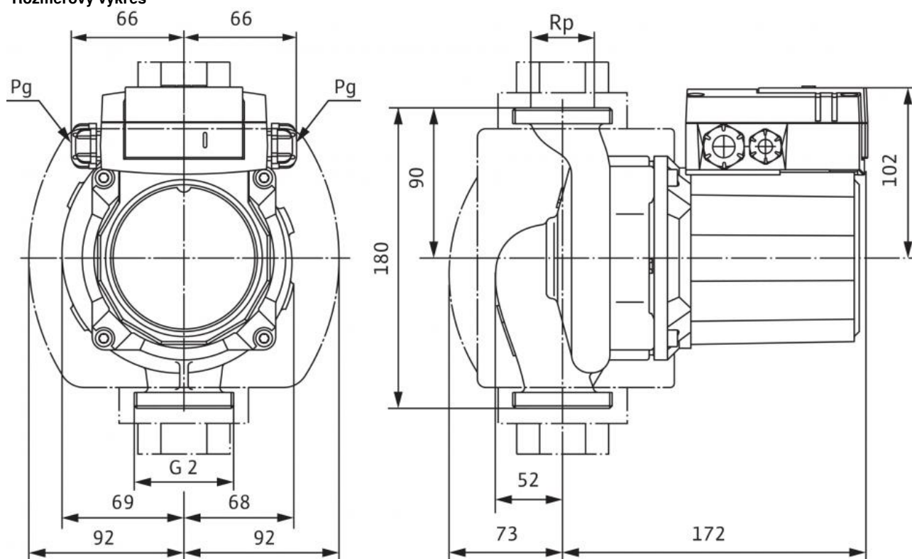
Rozmerový výkres
