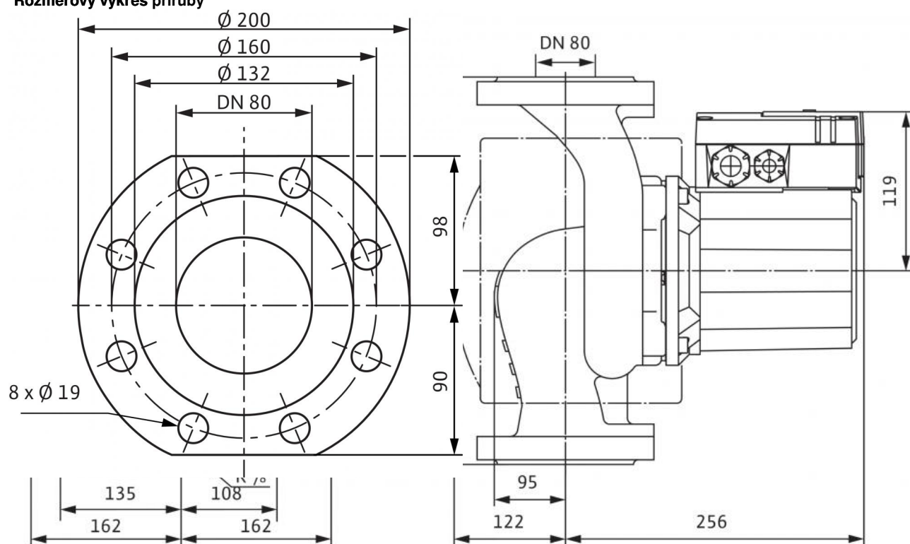
Rozmerový výkres príruby
