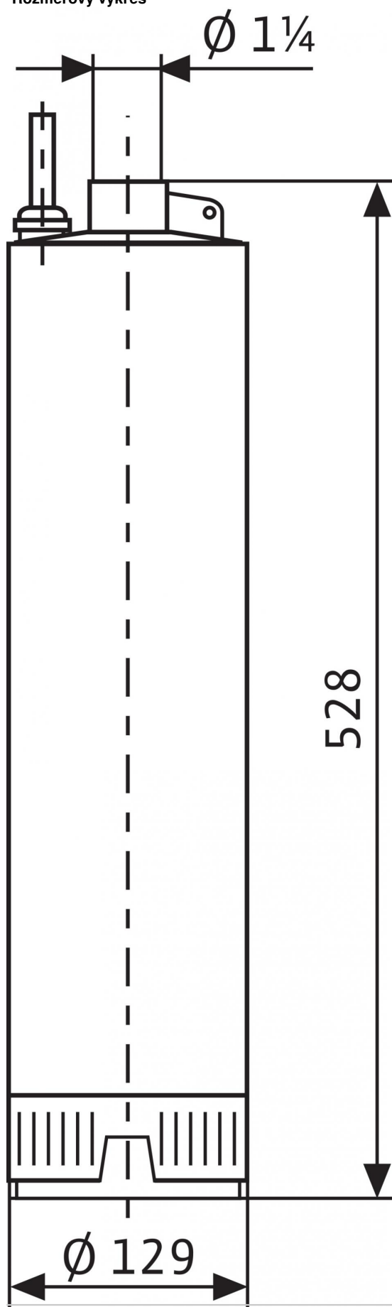
Rozmerový výkres
