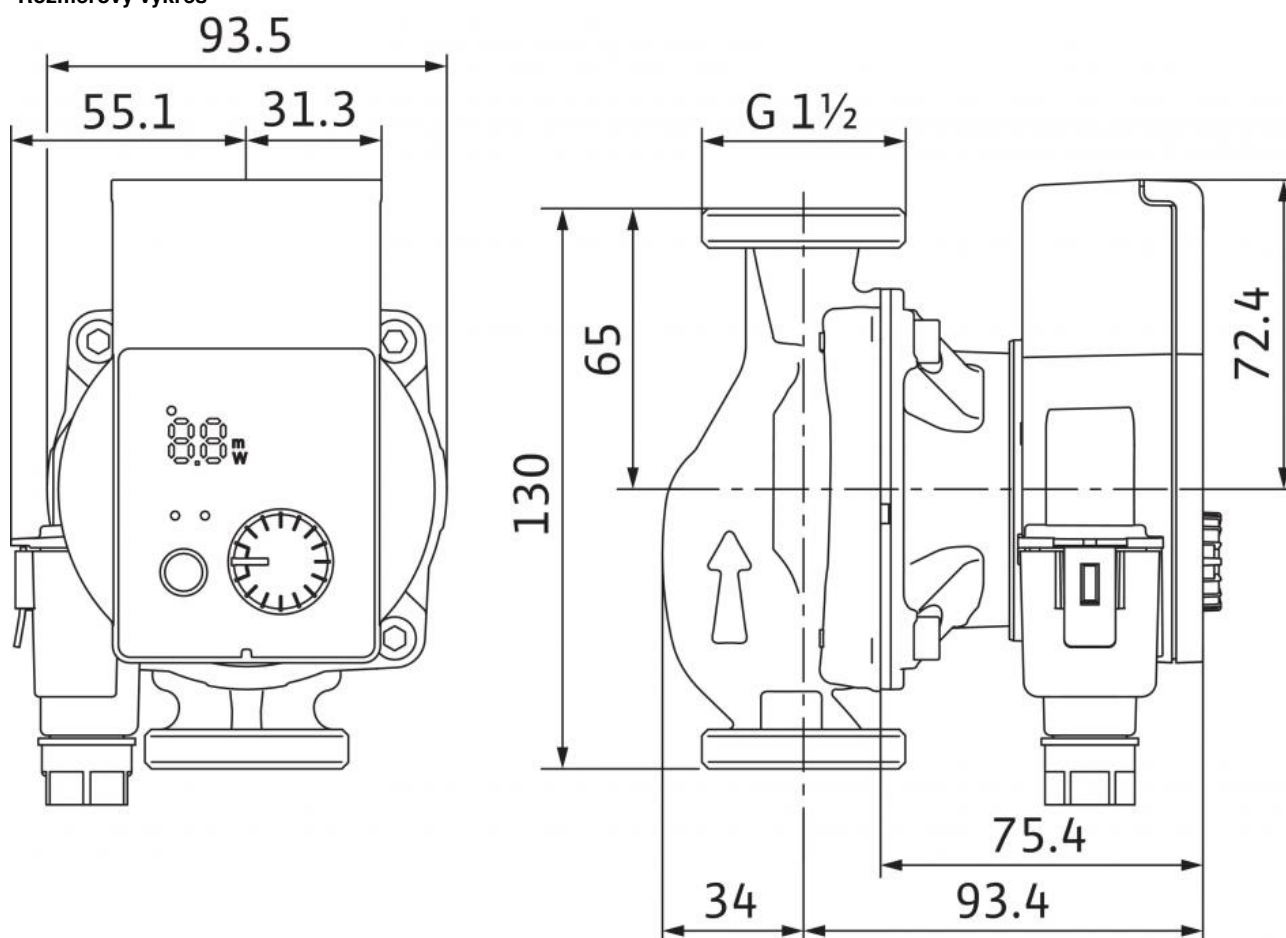
Rozmerový výkres
