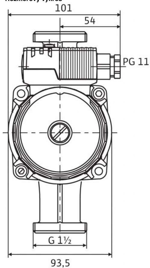
Rozmerový výkres
