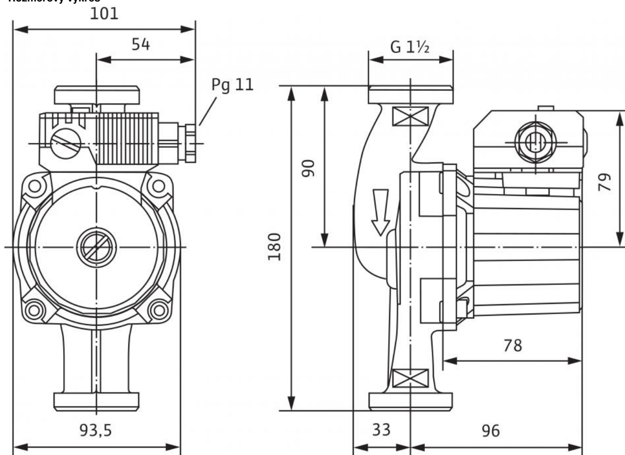
Rozmerový výkres
