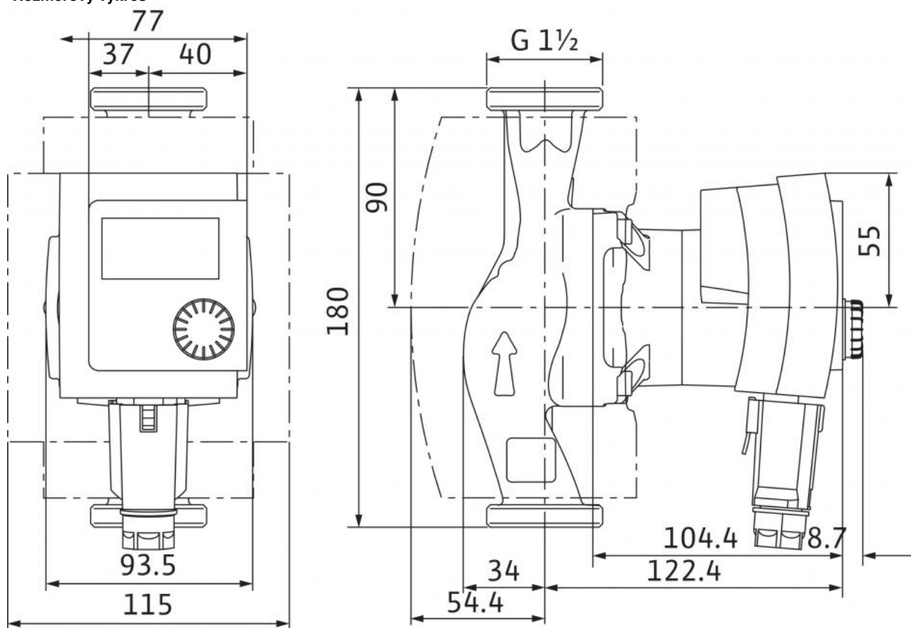
Rozmerový výkres
