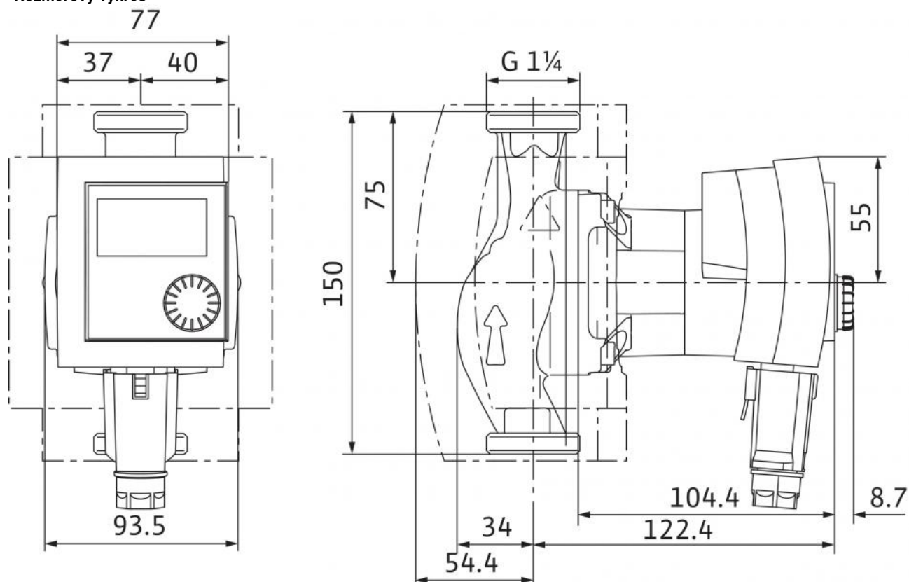
Rozmerový výkres
