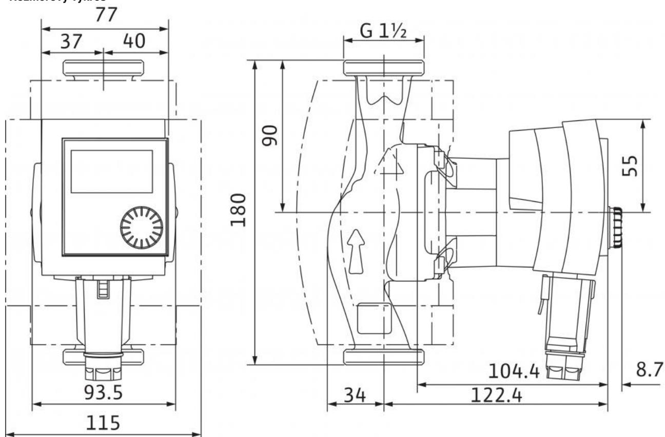
Rozmerový výkres
