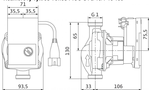
Rozmerový výkres Yonos PICO STG 15/1-13 130
